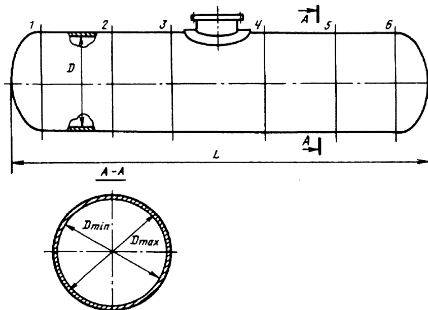
Эскиз № 1 к разделу "6. Карта измерений корпуса сосуда"
